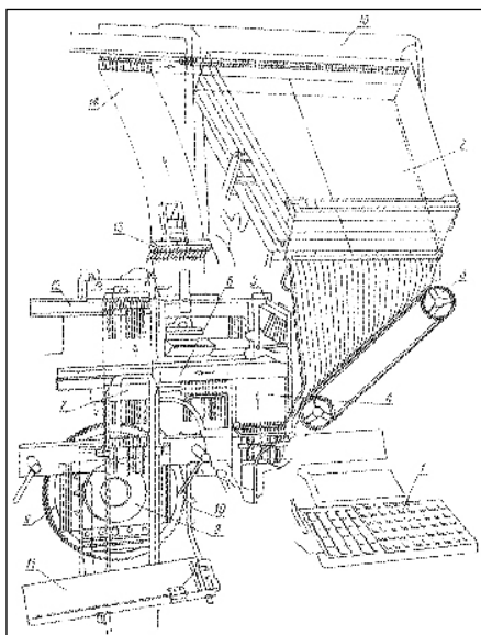
1. Linotyp – schemat pracy na podstawie dokumentacji J. Czopowicza 2008
