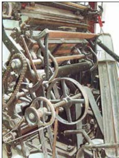
3. Linotyp – widok od strony napędu – stan przed remontem – fot. J. Czopowicz 2008
