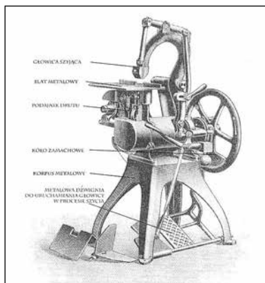
11. Zszywarka introligatorska do ruchu ręcznego schemat na podstawie dokumentacji – fot. J. Czopowicz 2008
