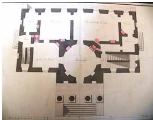
4. Rzut parteru wg proj. z pracowni D. Merliniego – 1872 rok.
