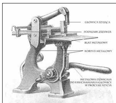
13. Zszywarka do szycia drutem – stan po remoncie – fot. J. Czopowicz 2008
