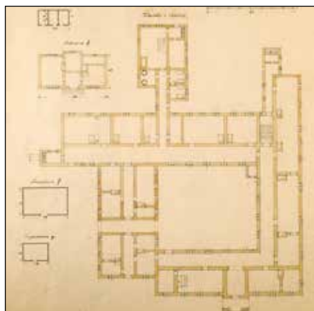
4. Biała Podlaska, szpital i klasztor SS Szarytek. Pomiar klasztoru z ok. 1880 r., op. przez M. Pawłowskiego.
